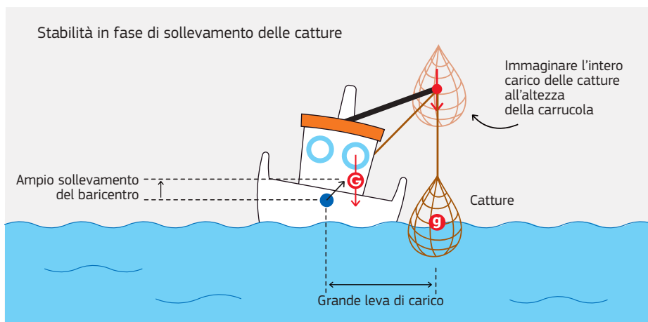
VI-11. Sollevamento dall'albero di carico.
